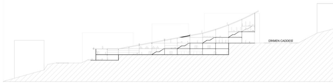
A-A KESİT 1/200
